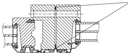
Snitt D-D
